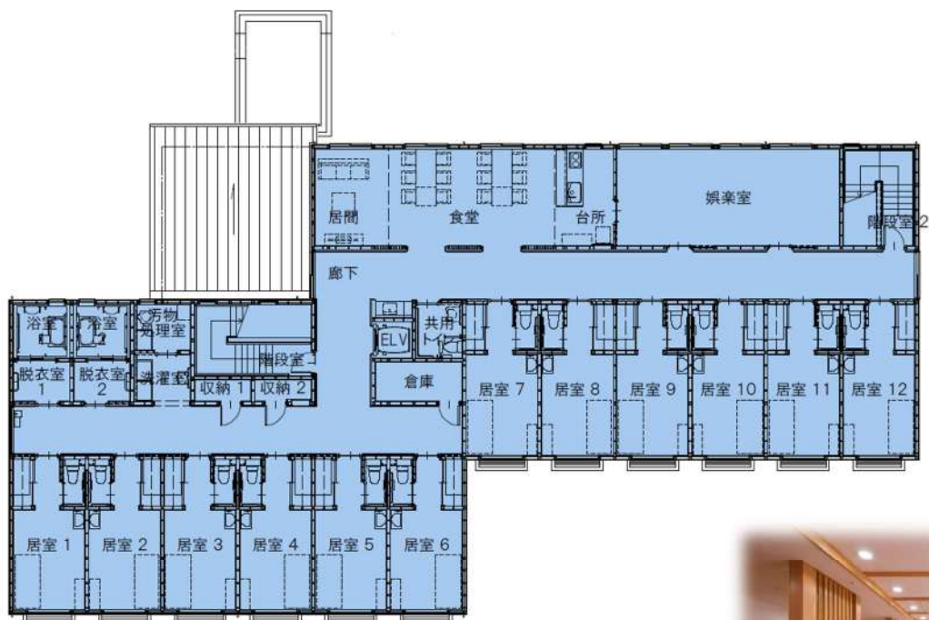
2階 平面図
